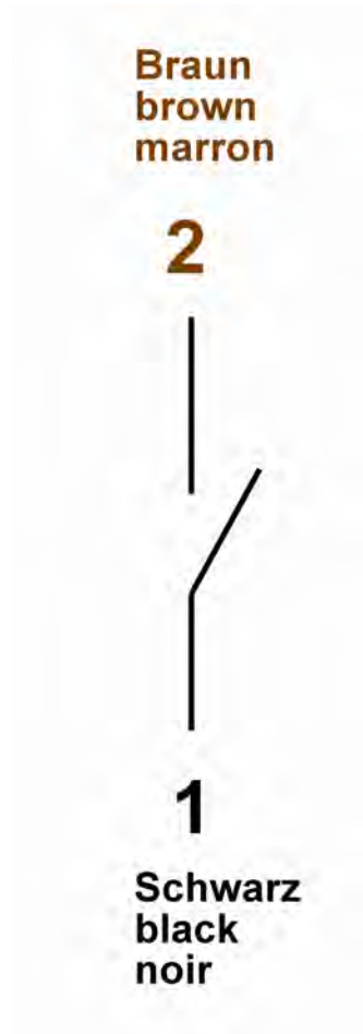
Abb. 20: Zustand des Kontakts bei Gerät ohne Durchfluss
