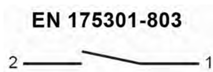
Abb. 13: Zustand des Kontakts bei Gerät ohne Durchfluss
