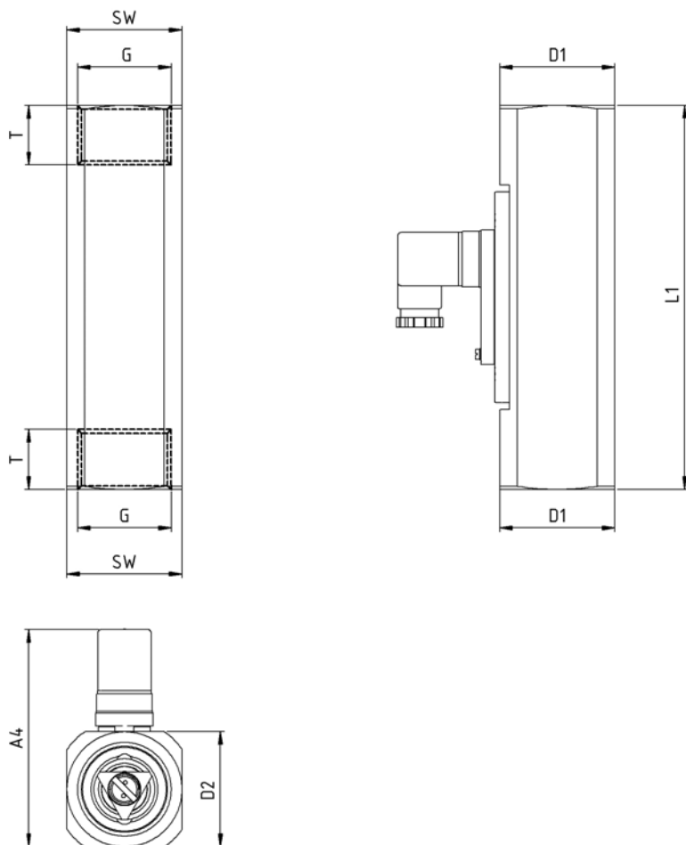
Abb. 65: Typ DUM-220 ATEX u. DUM-250
