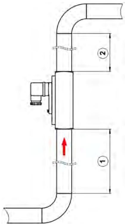
Abb. 6: Beruhigungsstrecken
