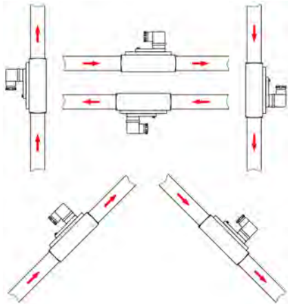
Abb. 5: Einbauposition/Durchflussrichtung
