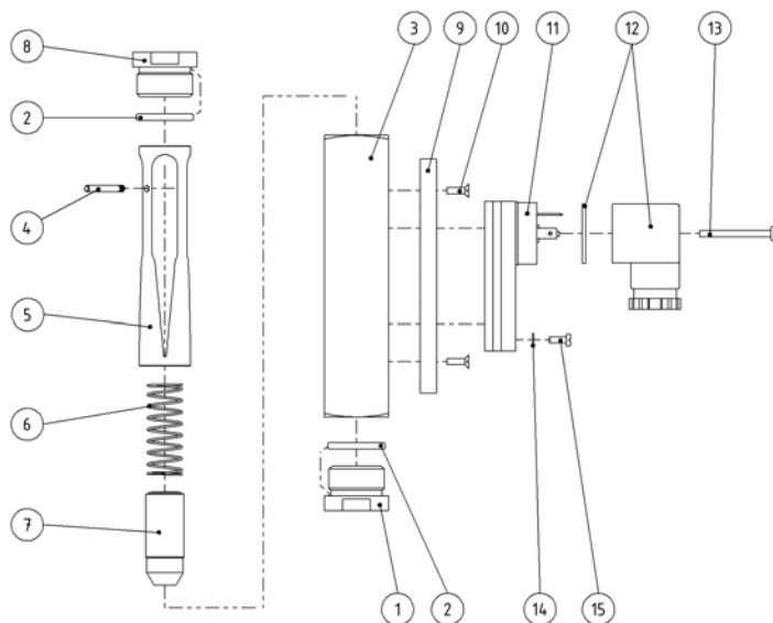
Abb. 66: Typ DUM-55
