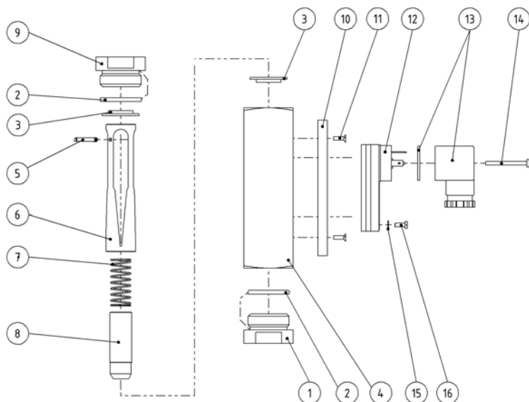
Abb. 67: Typ DUM-90
