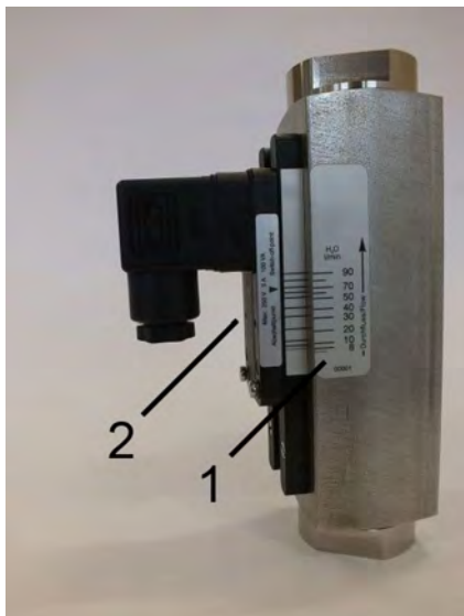
Abb. 1: Strömungswächter DUM
