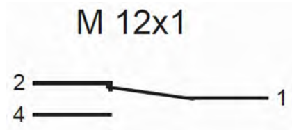
Abb. 19: Zustand des Kontakts bei Gerät ohne Durchfluss
