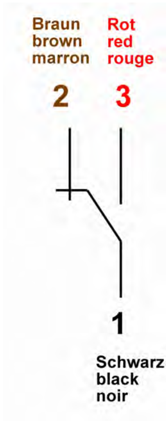
Abb. 21: Zustand des Kontakts bei Gerät ohne Durchfluss
