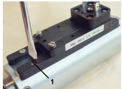
Abb. 60: Führungsleiste lösen
