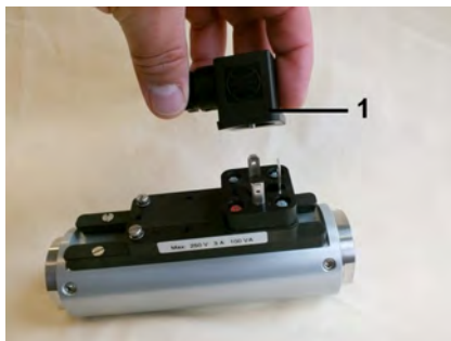
Abb. 58: Steckerdose abziehen
