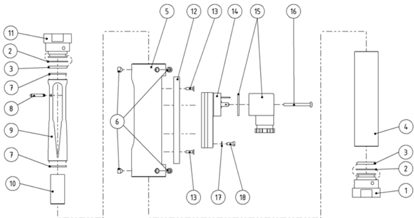
Abb. 68: Ersatzteilzeichnung
