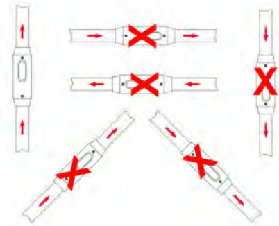
Abb. 5: Einbauposition/Durchflussrichtung
