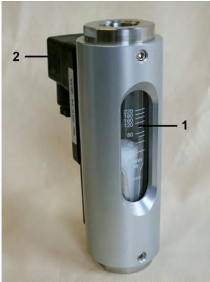
Abb. 1: Strömungswächter DWG-L
