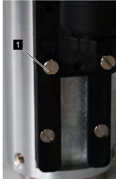
Abb. 33: Feststellschrauben lösen
