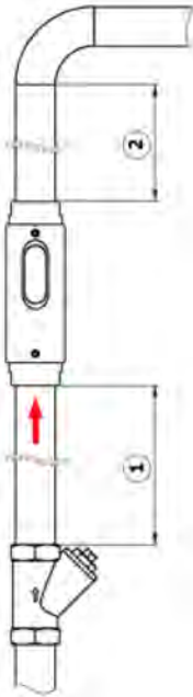
Abb. 7: Schmutzfänger
