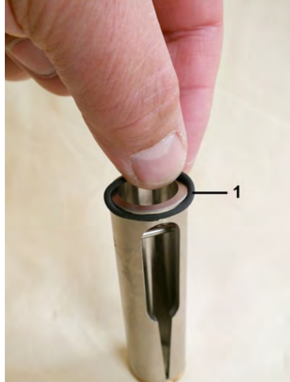
Abb. 44: O-Ring (Schlitzdüsenzentrierung)
