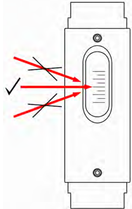
Abb. 34: Messskala ablesen
