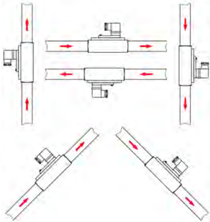
Abb. 5: Einbauposition/Durchflussrichtung
