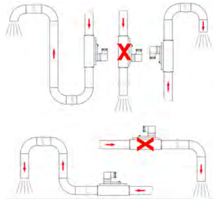
Abb. 7: Freier Auslauf
