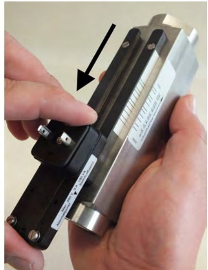
Abb. 64: Schaltkontakt aus Führung schieben
