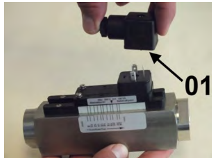
Abb. 62: Steckerdose abziehen
