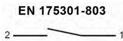
Abb. 13: Zustand des Kontakts bei Gerät ohne Durchfluss
