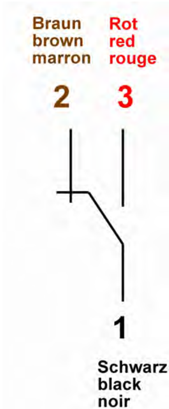
Abb. 21: Zustand des Kontakts bei Gerät ohne Durchfluss
