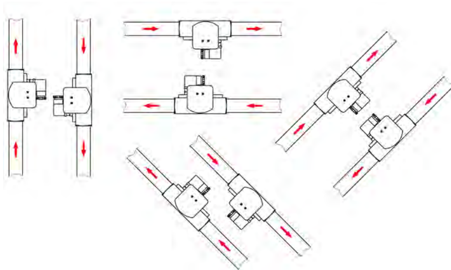
Abb. 6: Einbauposition/Durchflussrichtung
