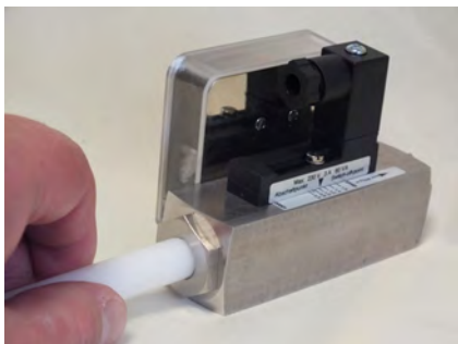
Abb. 61: Gängigkeit prüfen
