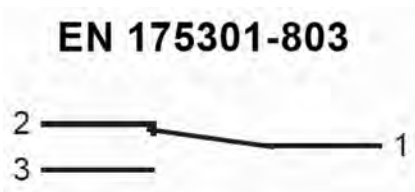
Abb. 16: Zustand des Kontaktes bei Gerät ohne Durchfluss
