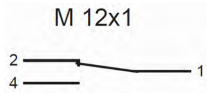
Abb. 20: Zustand des Kontaktes bei Gerät ohne Durchfluss
