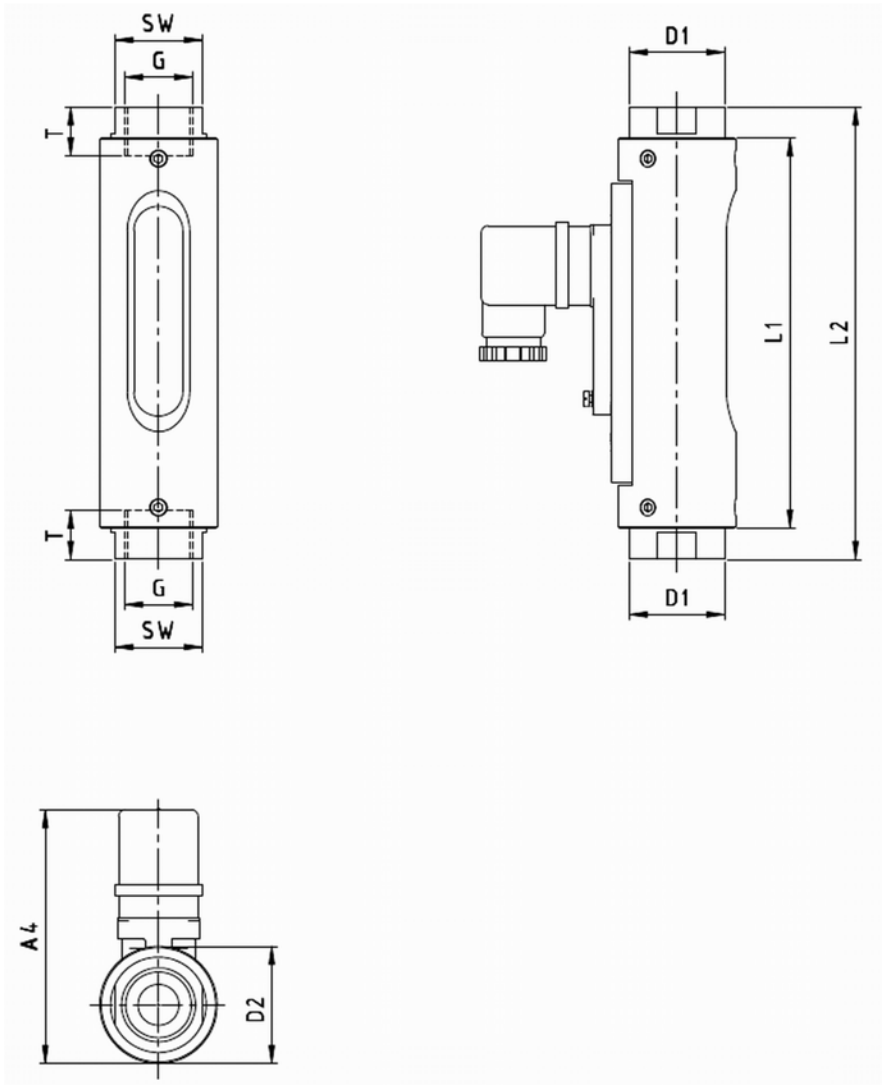
Fig. 70: Dimension sheet
