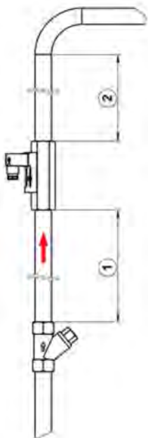
Fig. 8: Strainer
