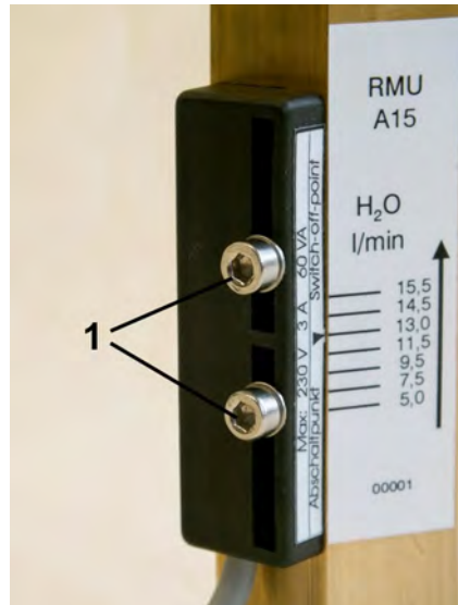
Abb. 19: Feststellschrauben lösen (Beispielskala)
