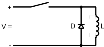
Abb. 14: Beispiel 1
