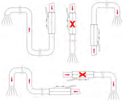
Abb. 7: Freier Auslauf
