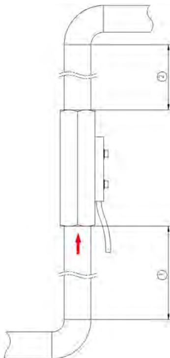
Abb. 6: Beruhigungsstrecken
