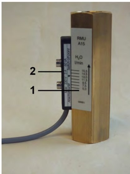
Abb. 1: Strömungswächter RMU-A
