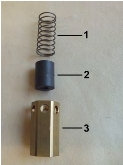
Abb. 27: Innenteile
