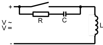
Abb. 15: Beispiel 2
