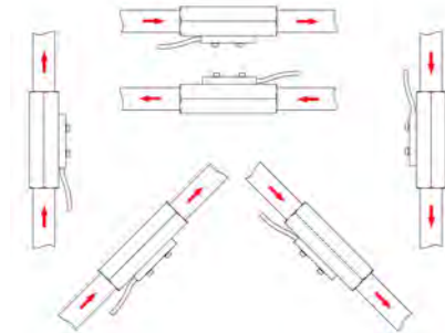
Abb. 5: Einbauposition/Durchflussrichtung
