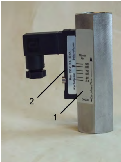
Abb. 1: Strömungswächter RVM/U-L2
