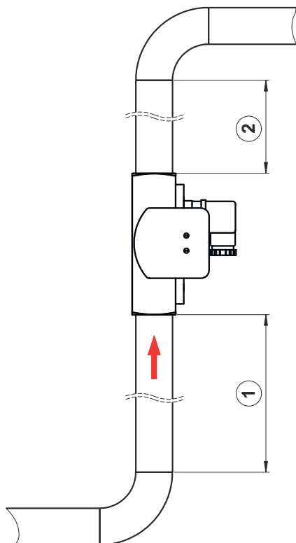
Fig. 9: Strainer
