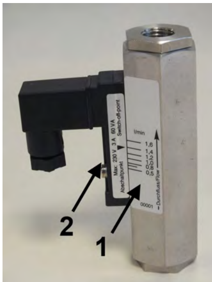
Abb. 1: Strömungswächter DKM-2
