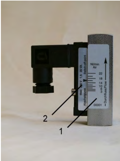
Abb. 1: Strömungswächter RVM/U-L4
